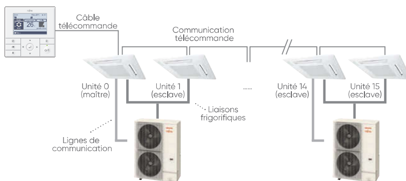
Télécommande filaire
